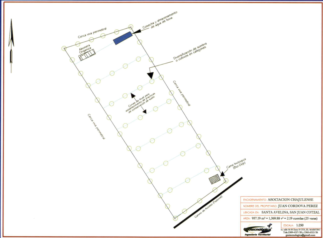
Figura 8. Plano ilustrativo de los componentes aplicables en la parcela de café menor a 15 cds, del Sr. Juan Córdoba Pérez.
